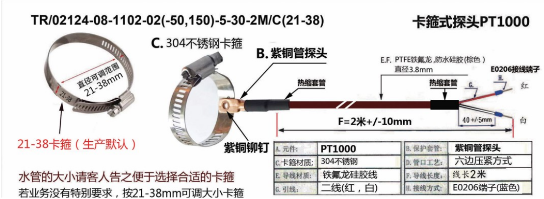
图二 卡箍式 PT1000 尺寸图 (图片供参考, 以实物为准)
